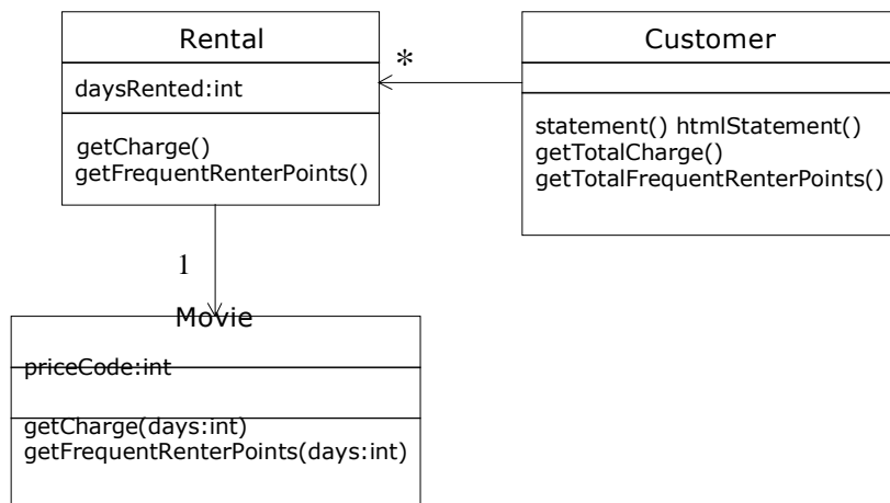
图 1.13 本节所讨论的两个函数被移到 Movie class 内之后系统的 class diagram。
