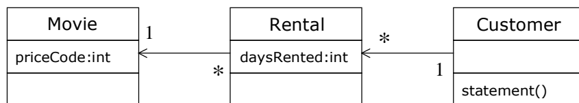
图 1.1 本例一开始的各个 classes。此图只显示最重要的特性。图中所用符号是 UML（Unified Modeling Language，统一建模语言，[Fowler, UML]）。
